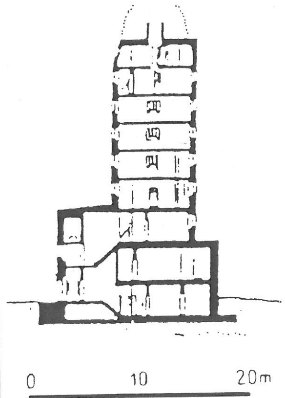
Przekrój wieży obserwacyjnej wg Marcina Dudka
